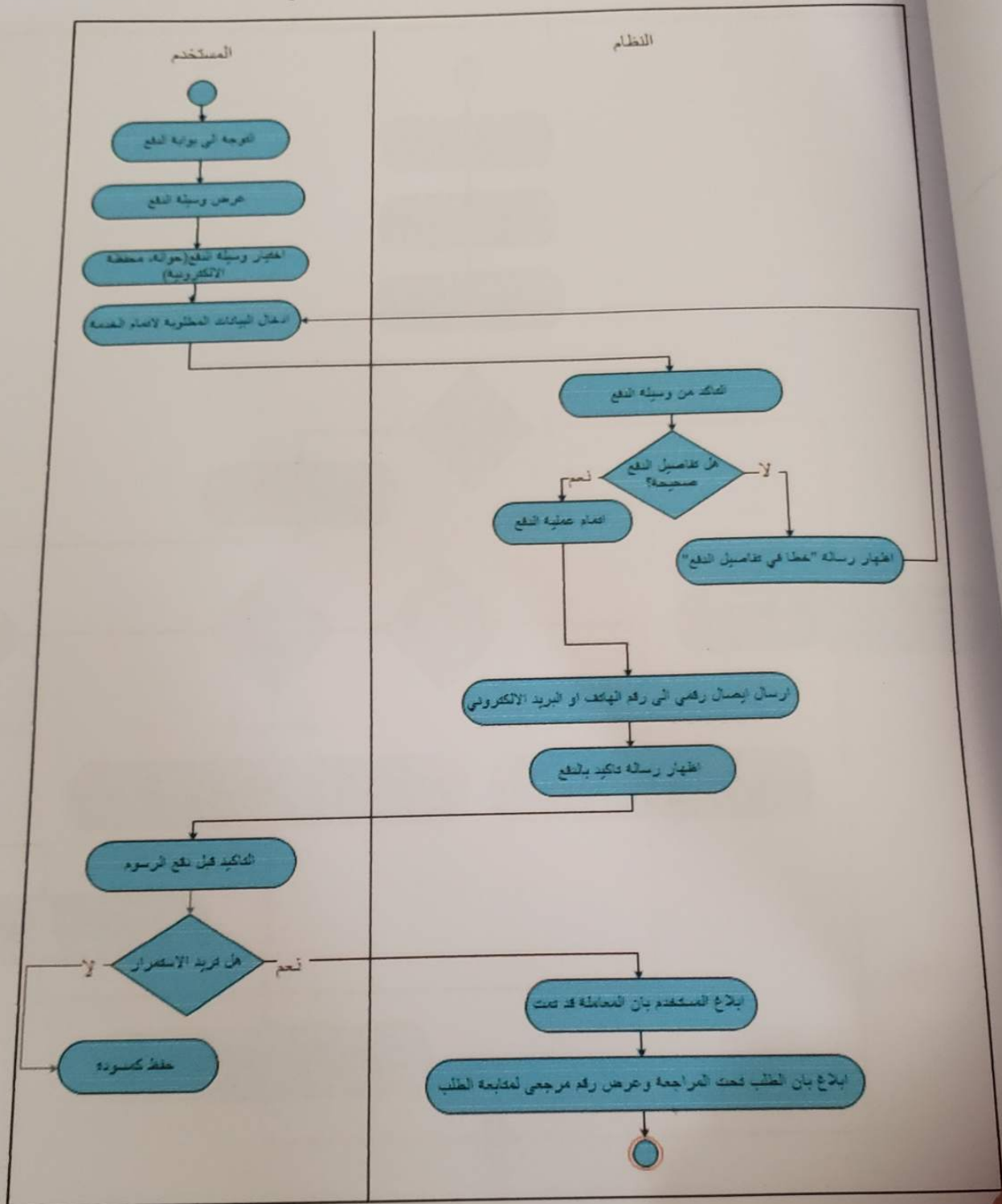
الشكل (3.11) مخطط النشاط للدفع
