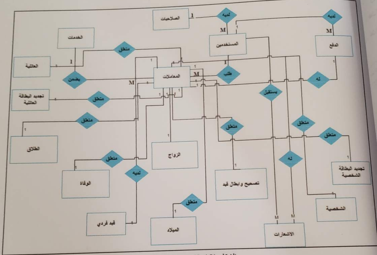
الشكل (3.18) مخطط العلاقات
