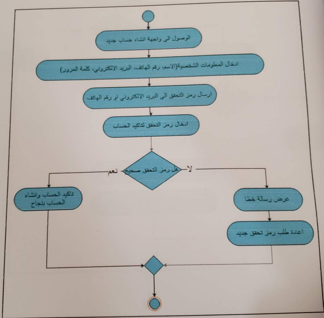
الشكل (3.8) مخطط النشاط لإنشاء حساب
