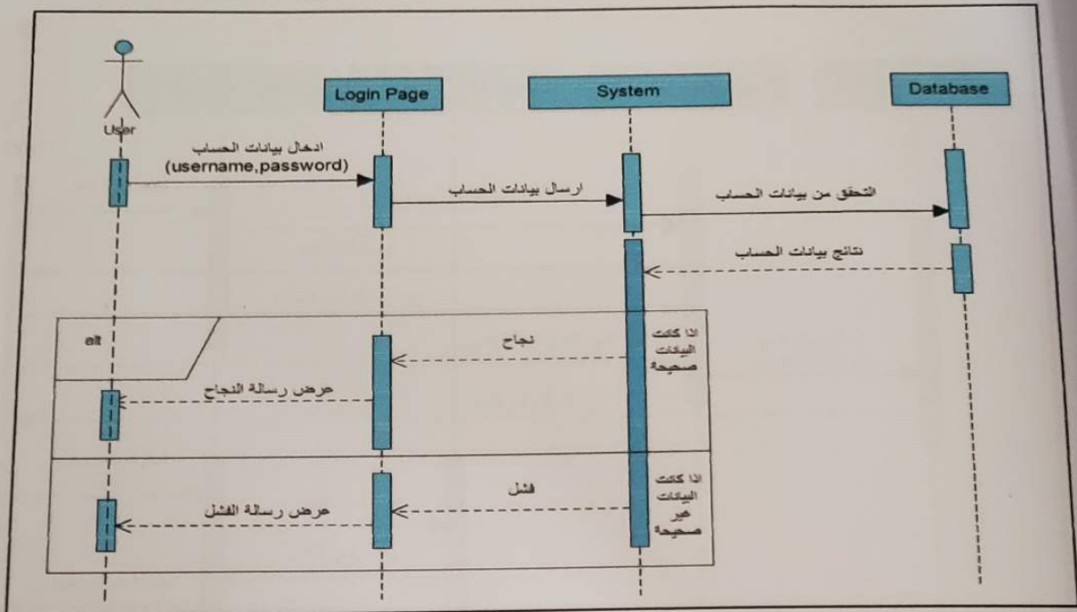
الشكل (3.4) مخطط التسلسل لتسجيل الدخول
