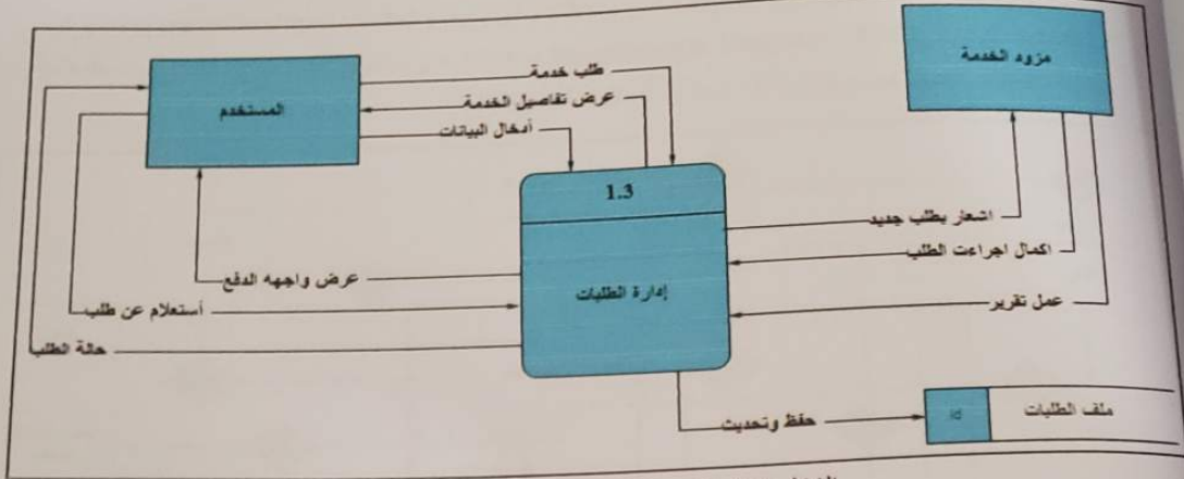
الشكل (3.16) مخطط تدفق البيانات إدارة الطلبات
