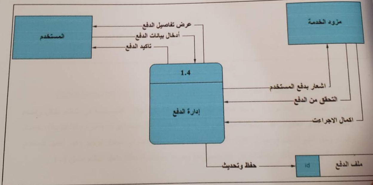
الشكل (3.17) مخطط تدفق البيانات إدارة الدفع
