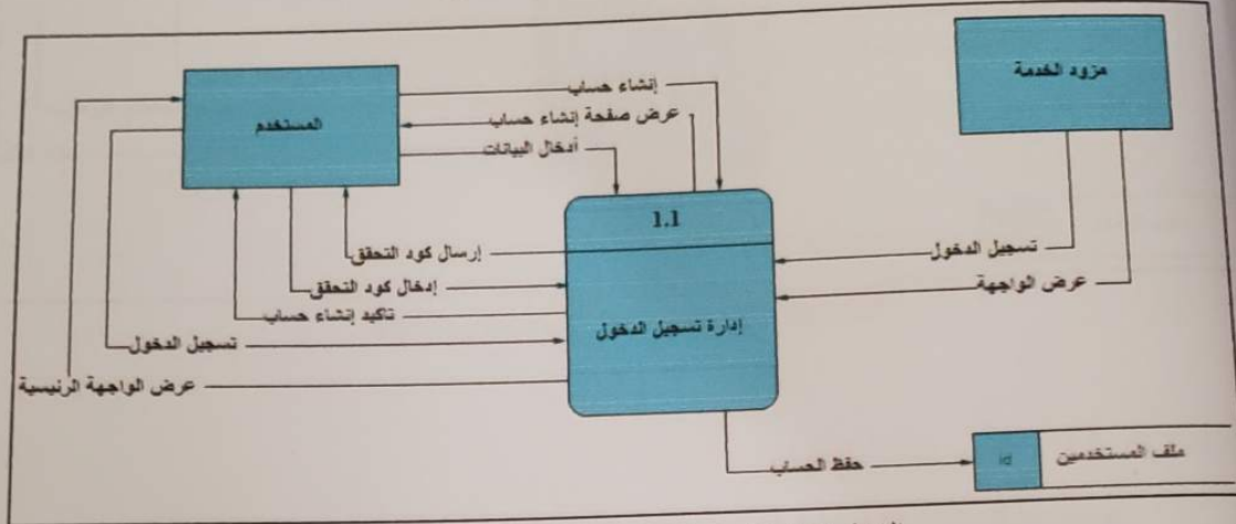
الشكل (3.14) مخطط تدفق البيانات لتسجيل الدخول
