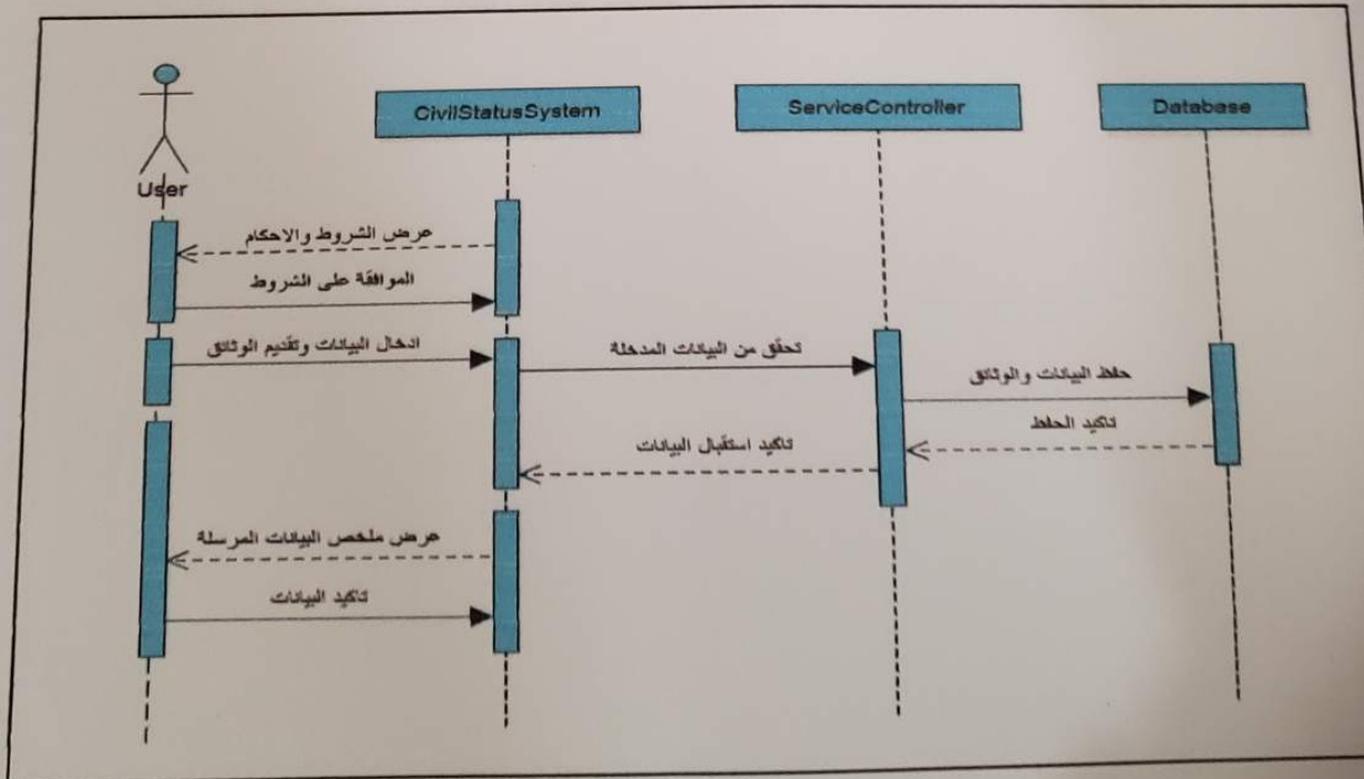
الشكل (3.5) مخطط التسلسل لإدخال البيانات
