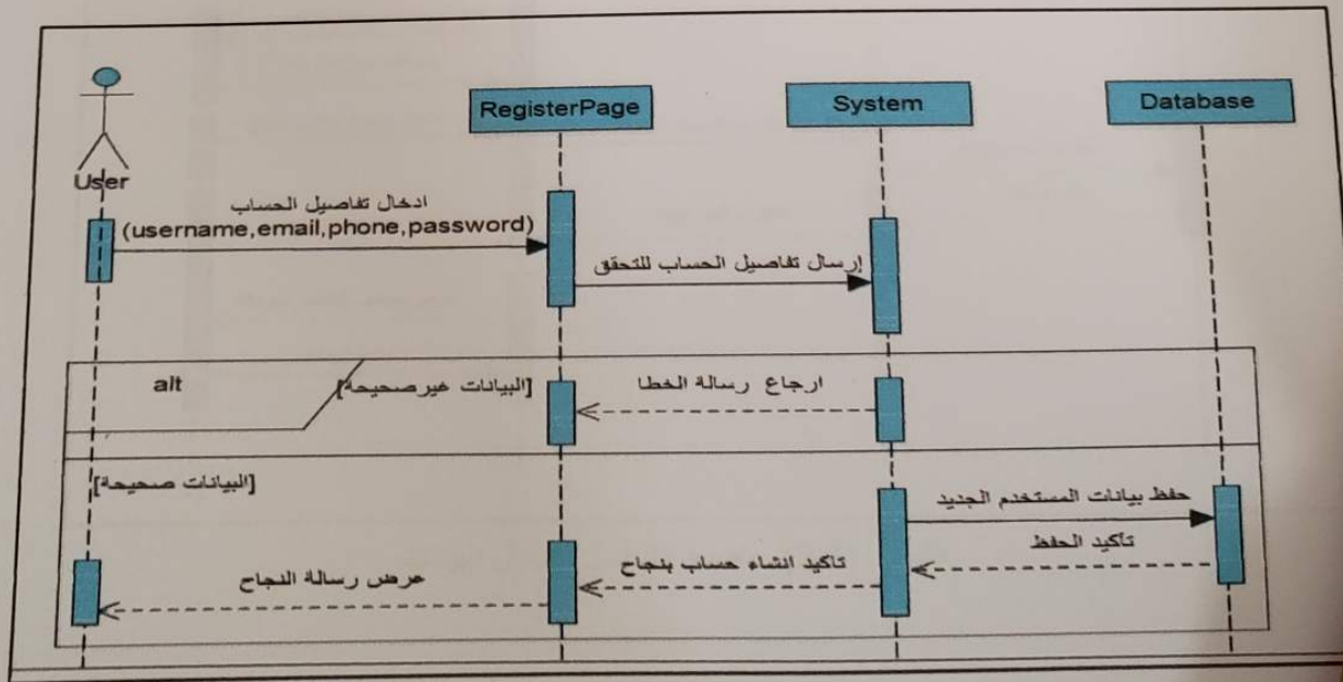
الشكل (3.3) مخطط التسلسل لإنشاء حساب
