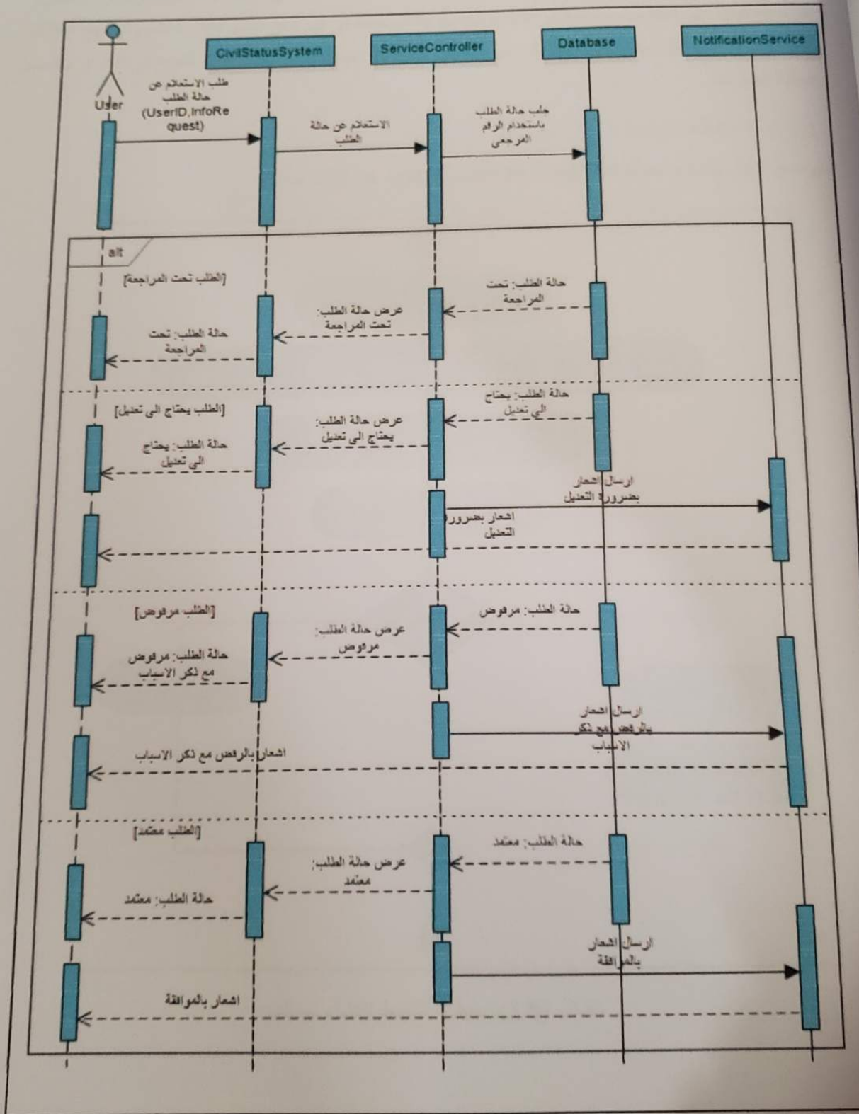
الشكل (3.7) مخطط التسلسل للاستعلام عن حالة طلب
