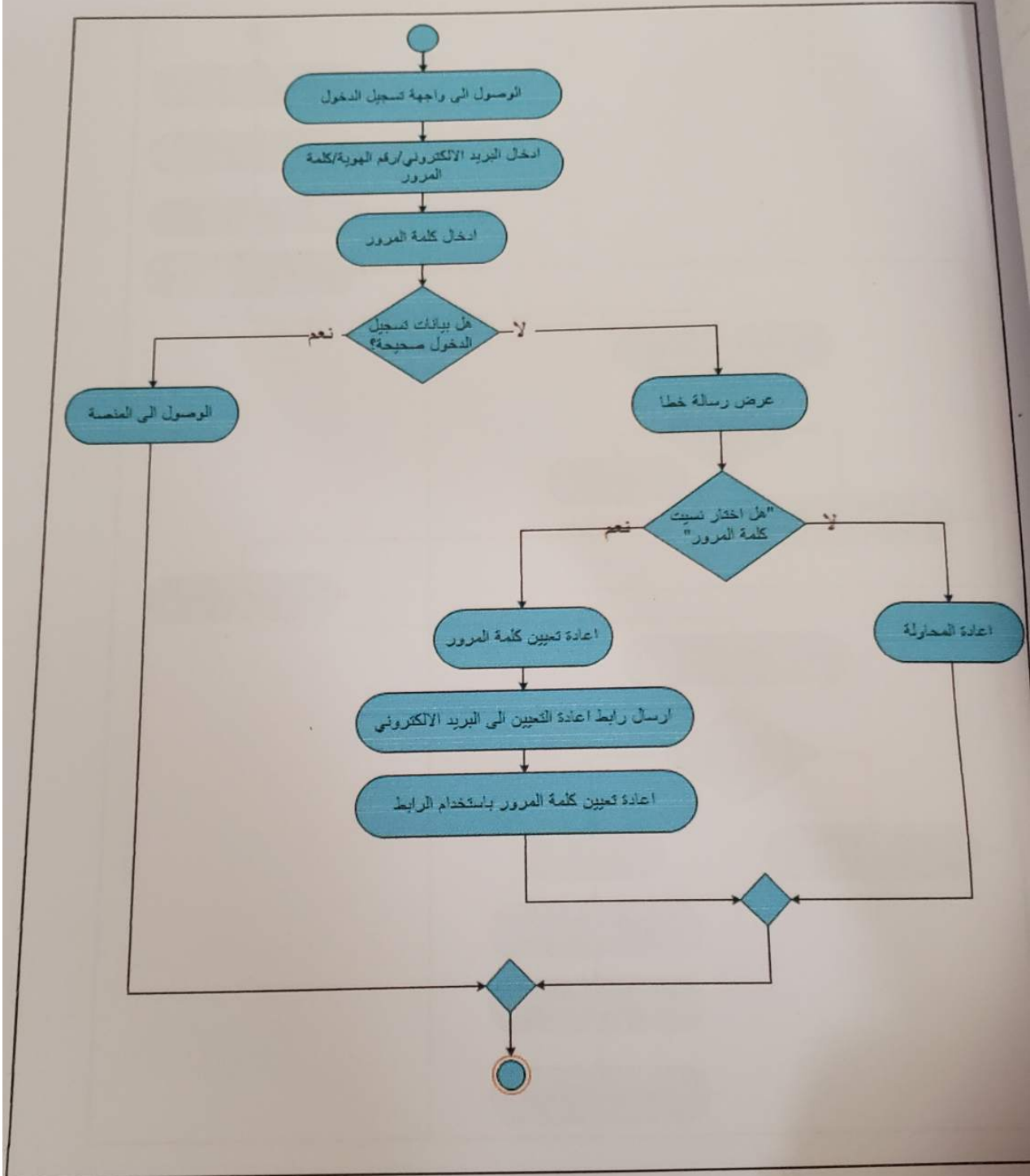
الشكل (3.9) مخطط النشاط لتسجيل الدخول
