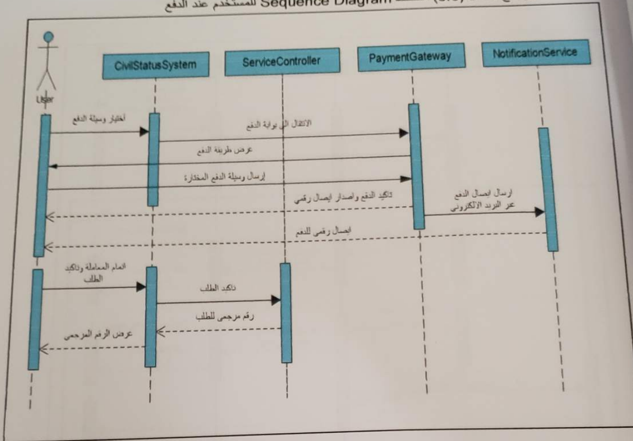
الشكل (3.6) مخطط التسلسل للدفع
