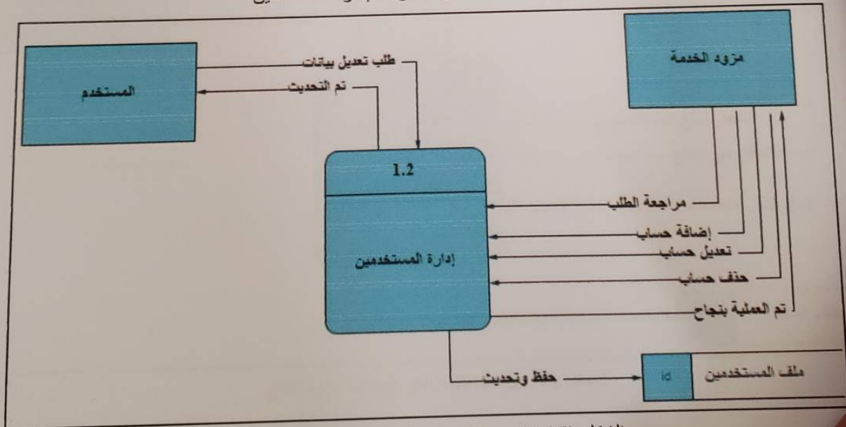
الشكل (3.15) مخطط تدفق البيانات لإدارة المستخدمين
